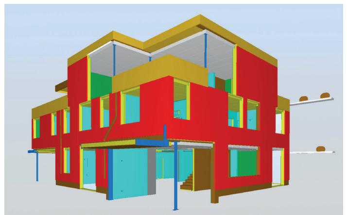
Illustration 20: Modèle de bâtiment réalisé avec la technologie BIM
